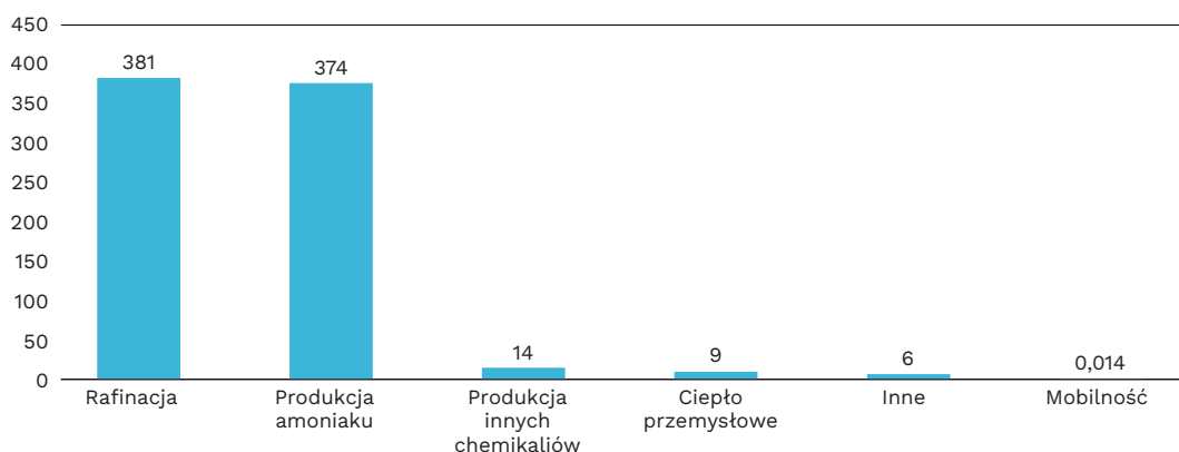
Wykres 5. Popyt na wodór w Polsce w 2022 r. w podziale na zastosowanie końcowe (w tys. t rocznie)
